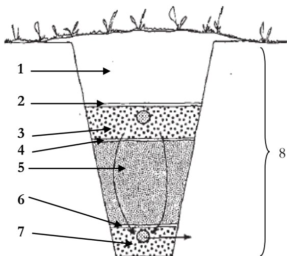
Markbädd (sektion).
